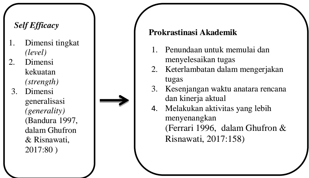
Gambar 1 Kerangka Konseptual
