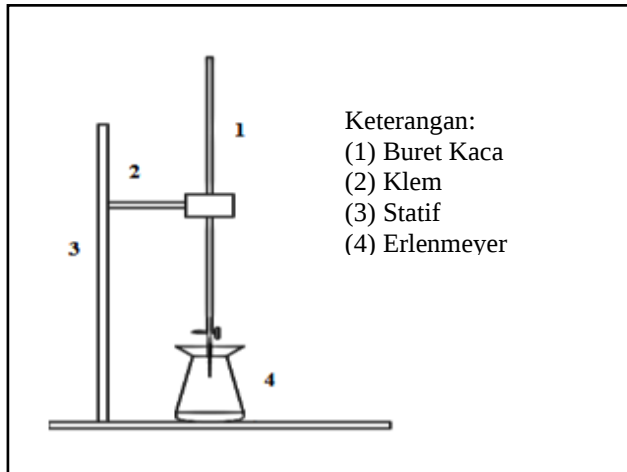
Gambar 4. Rangkaian Alat Proses Titrasi (Widayanti E, 2025)
