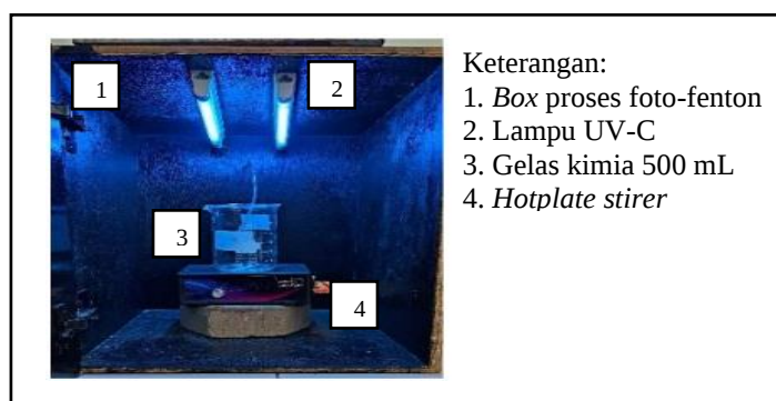
Gambar 2. Rangkaian Alat Proses Foto-Fenton (Adnan dkk., 2023)
