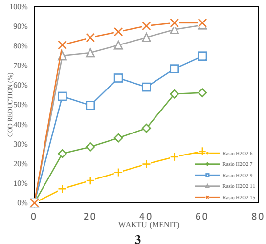
Gambar 6. Efisiensi penurunan COD berbagai rasio H_2O_2 /COD pada pH 3
