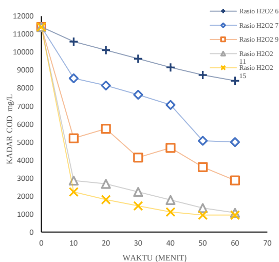
Gambar 5. Pengujian COD berbagai rasio H_2O_2 /COD pada pH
