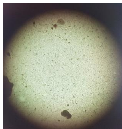
Gambar 1. Hasil Uji Homogenitas
