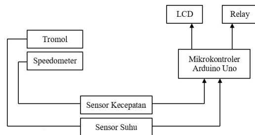
Gambar 11. Diagram Blok Sistem
