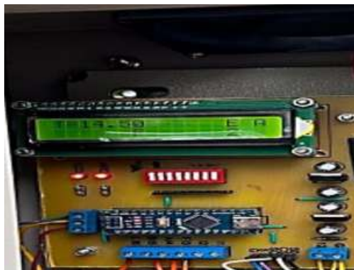
Gambar 3.2 Tampilan Awal LCD pada Incinerator
